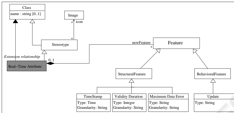
Figure 3: Abstract syntax of the «RealTimeAttribute» stereotype.
