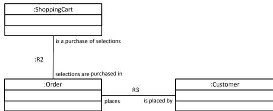
(a) \neg\text{Empty}(R2) \wedge \neg\text{Empty}(R3)
